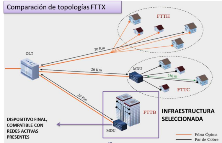
Figura 10. Infraestructura FTTX seleccionada. Fuente: elaboración propia (2017)
