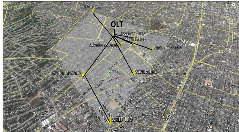
Figura 7. Topología estrella red GPON Fuente: Elaboración propia (2017)
