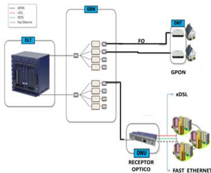
Figura 1. Topologías para conexión GPON, xdsl, pots, fast ethernet Fuente: Elaboración propia (2017)
