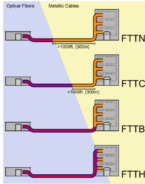
Figura 9. Tecnologías FTTX. Fuente: Cortés (2016)
