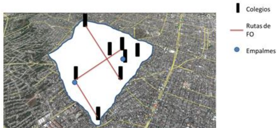
Figura 4. Líneas de FO recomendados Fuente: Elaboración propia (2017)
