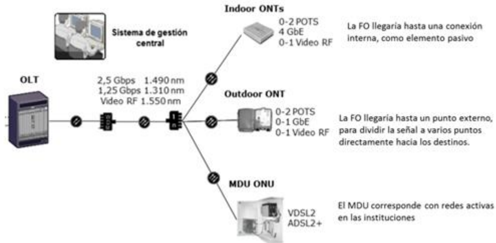
Figura 3. Elementos finales red GPON Fuente: Elaboración propia (2017)
