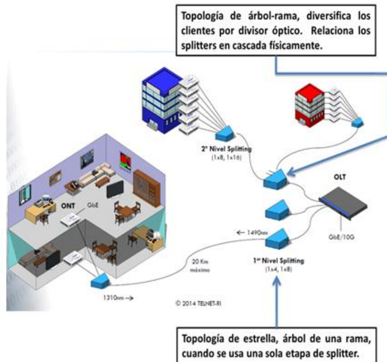
Figura 2. Topología de una red GPON Fuente: García (2014)
