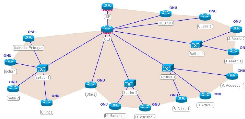
Figura 11. Topología de la Red. Fuente: Elaboración propia (2017)
