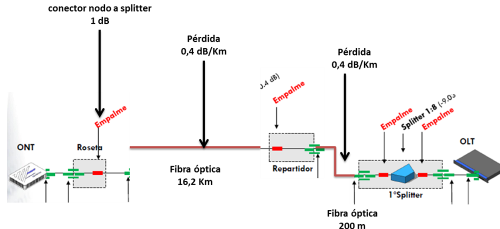
Figura 8. Elementos en la red GPON para interconexión del diseño Fuente: elaboración propia (2017)
