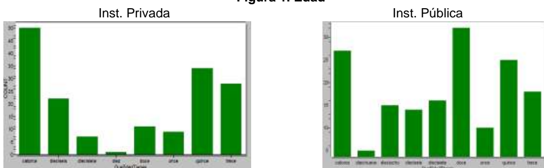
Figura 1. Edad
