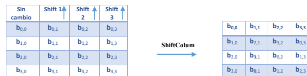
Figura 1. Función ShiftColumns
