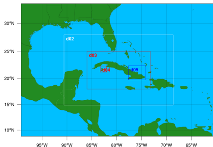
Fig. 2. Dominios confeccionados para el experimento descrito. Dominio de 1km de Gibara I (d05).
