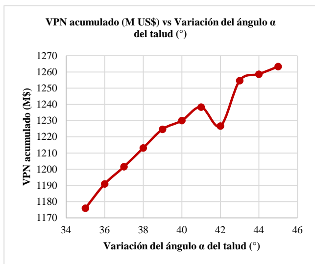
Figura 2. Variación del ángulo global del talud vs VPN acumulado. Fuente: Elaboración propia.
