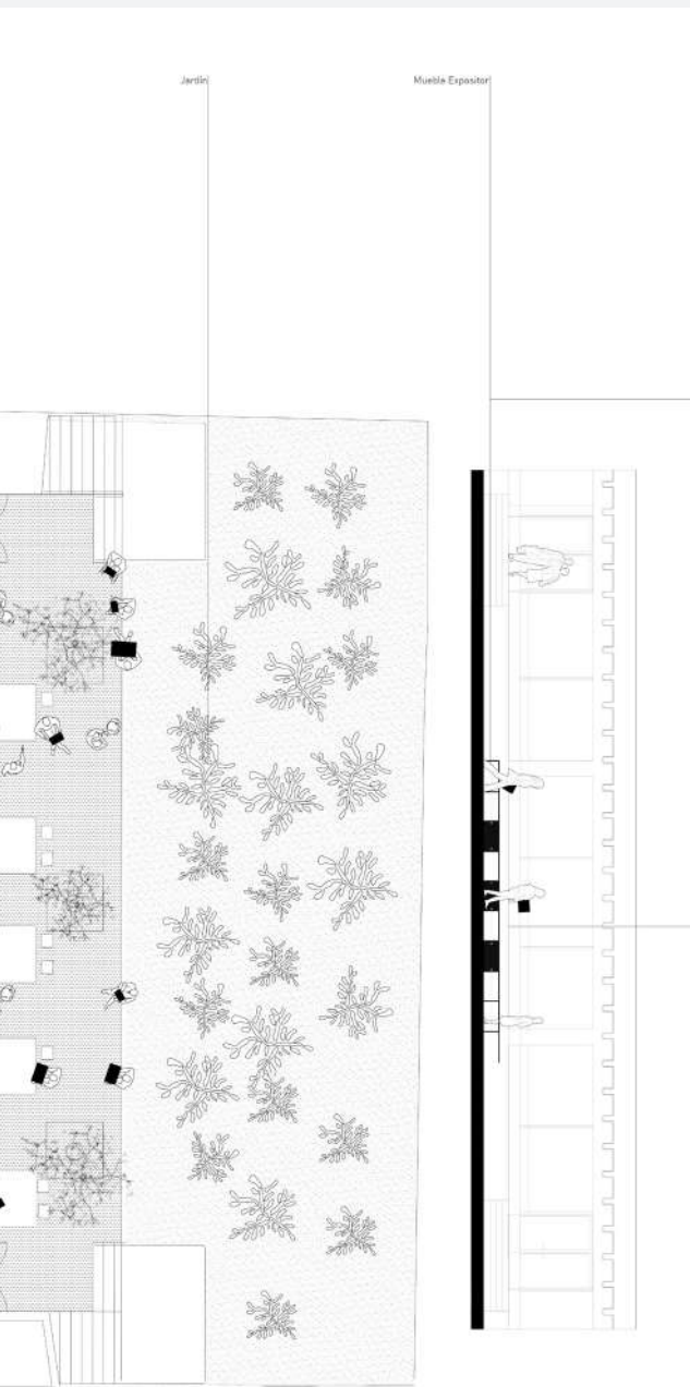
Alzado "Mueble Expositor"
