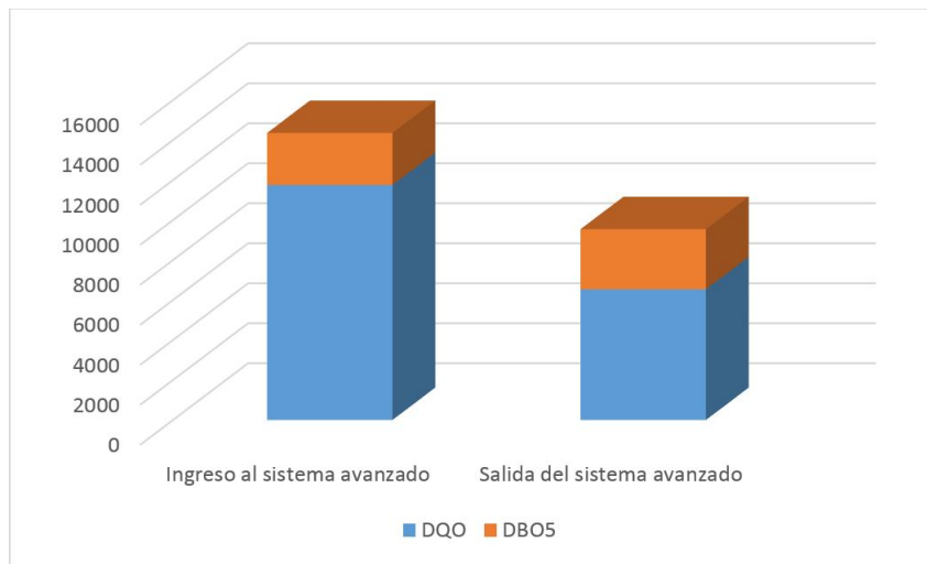
Figura 3. Gráfico de la disminución de DQO, aumento de la DBO 5 medidas en mg/L en la concentración óptima de reactivo Fenton modificado.
