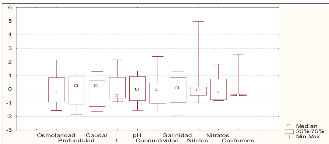
Figura 3. Box Plot con variables estandarizadas.
