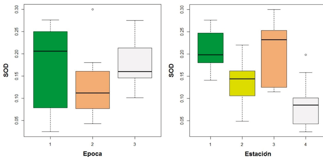
Figura 3. Diagrama de cajas para las diferentes épocas climáticas monitorizadas (1: época seca, 2: época lluviosa, 3: época transición) y las diferentes estaciones 1: Montenevado, 2: Charco Manso, 3: Casa Mía, 4: Puente Autopista) con respecto a la demanda de oxígeno por sedimentos
