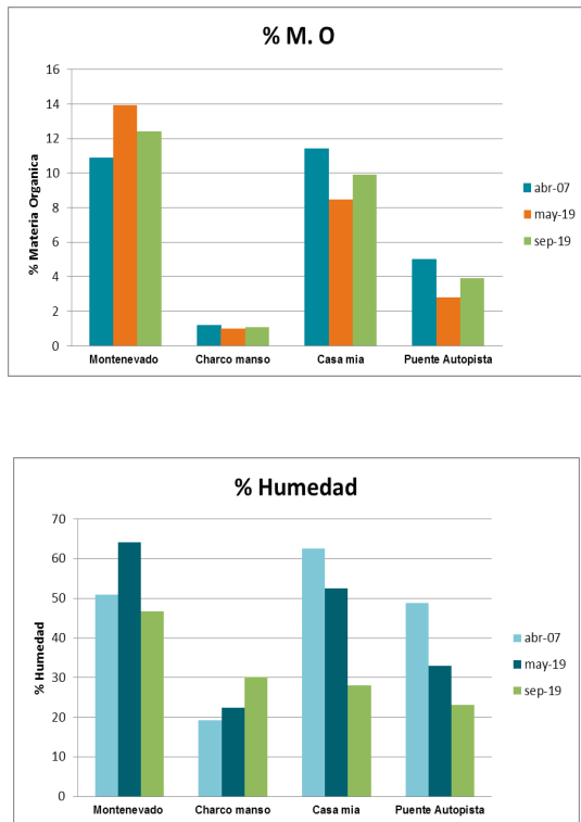
Figura 1. % MO y % humedad en las diferentes épocas y estaciones monitorizadas Fuente: autoría propia.
