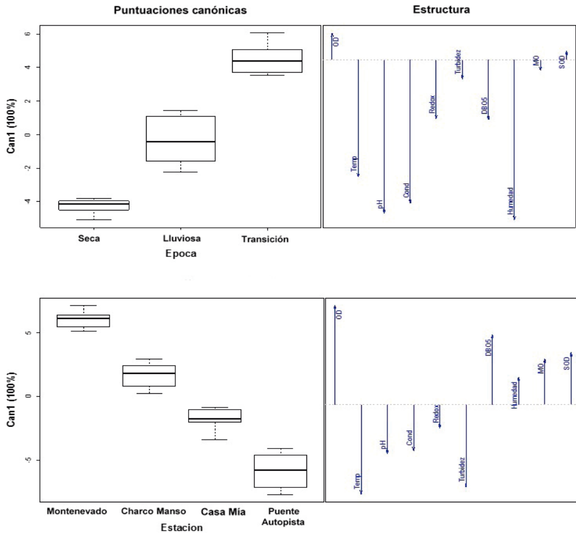
Figura 4. Análisis canónico discriminante de las diferentes variables para los factores época y estación
