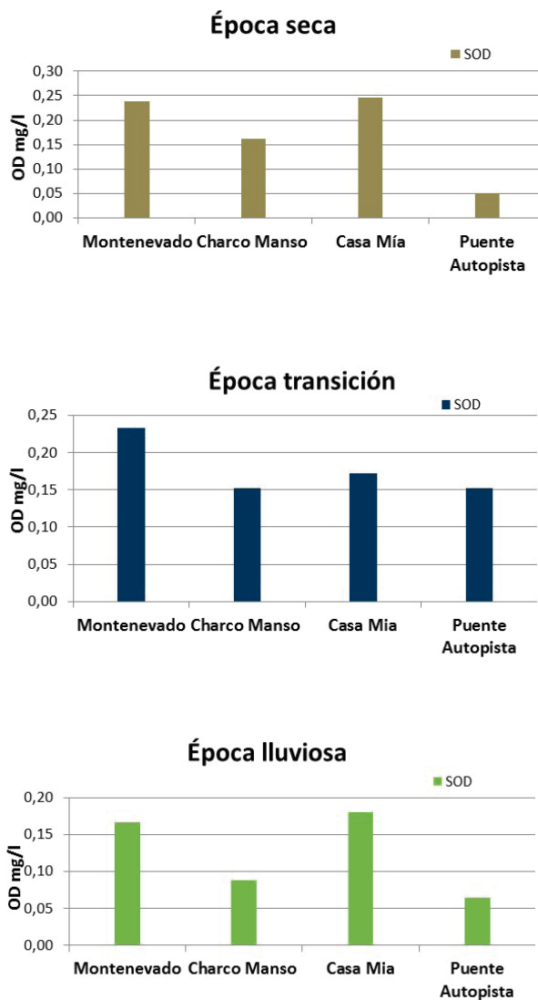
Figura 2. SOD en las diferentes estaciones y épocas monitorizadas
