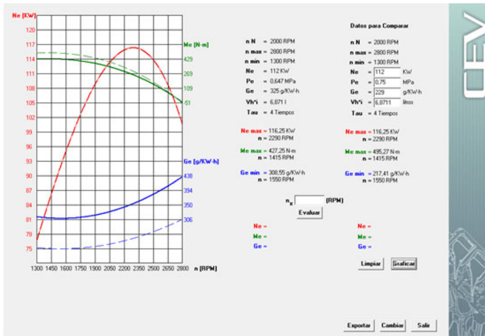
Figura. Comparación entre las características exteriores de velocidad de biodiesel y diésel.
