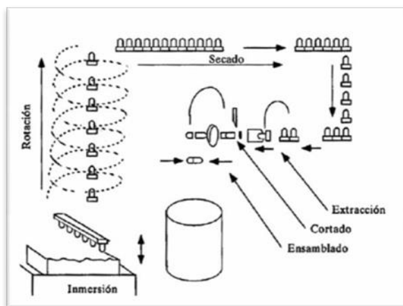
Figura 3. Esquema de proceso de fabricación de las cápsulas de gelatina dura
