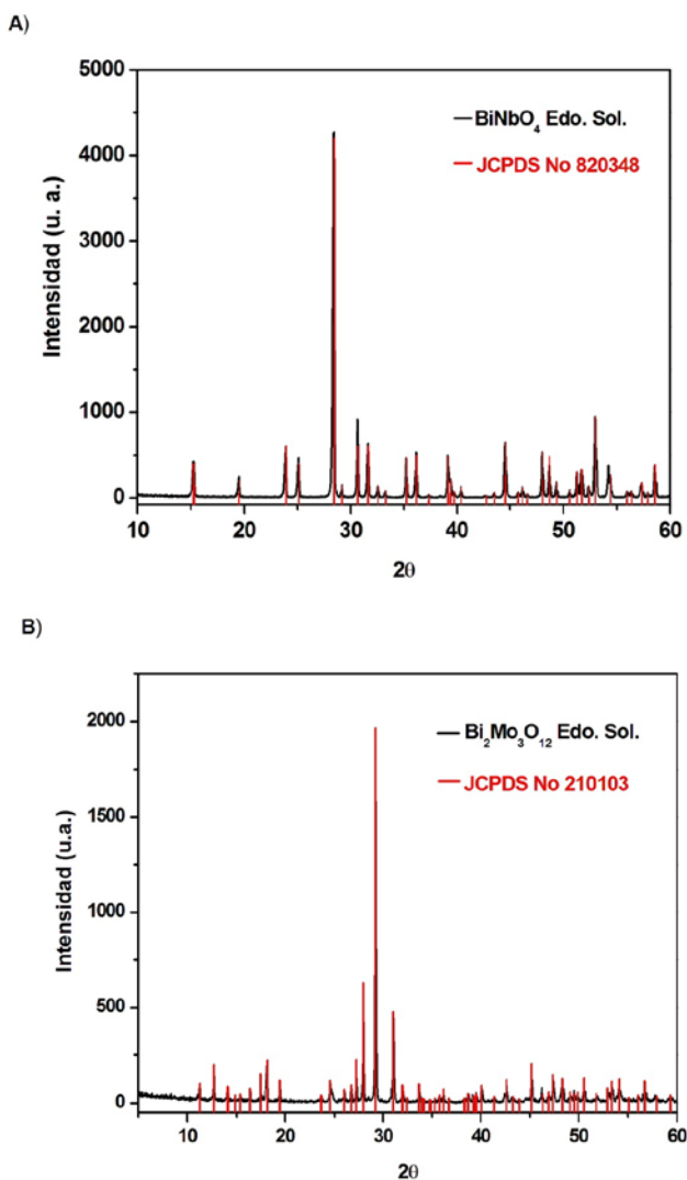
Figura 3. Difractogramas de los semiconductores sintetizados por reacción en estado sólido: a) \text{BiNbO}_4 y b) \text{Bi}_2\text{Mo}_3\text{O}_{12} .
