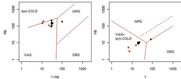
FIGURA 12. Diagramas de ambiente de discriminación tectónica de Pearce (1984) para muestras de edad Pérmica localizadas al occidente de La Plata y Pacarní - Huila.
