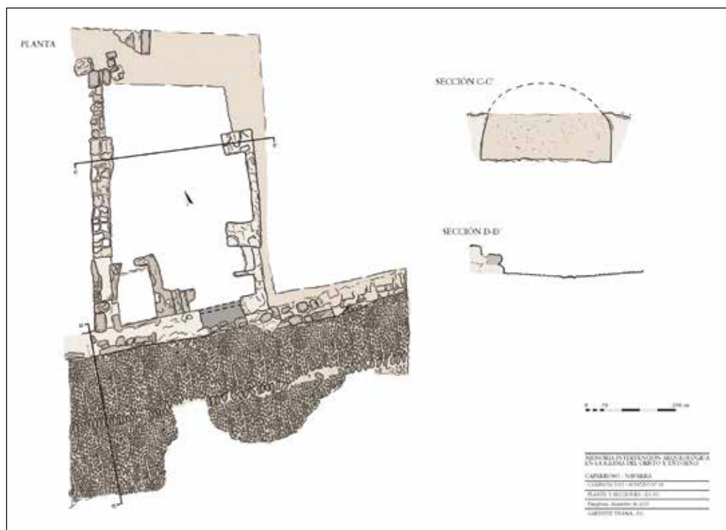
Planimetría del edificio excavado en 2015.
