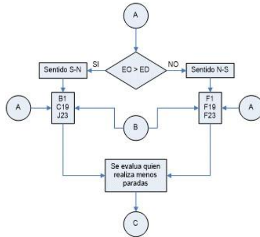
Figura 7. Diagrama de flujo para la selección de la ruta a partir de rutas posibles y del sentido Norte-Sur o Sur-Norte (Fuente: Propia)
