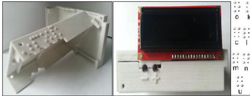
Figura 4. Interfaz Usuario – Dispositivo (Fuente: Propia)
