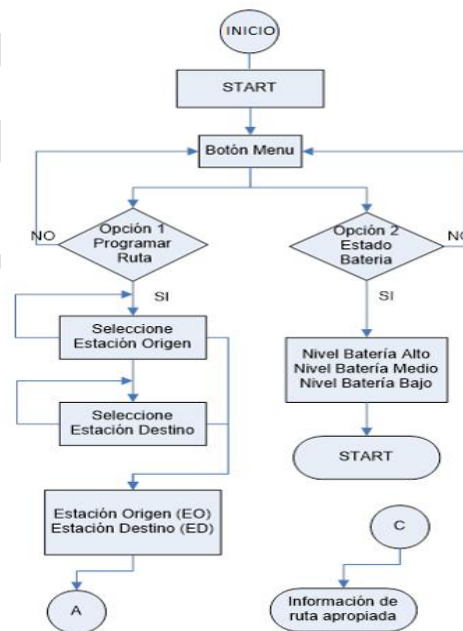
Figura 5. Diagrama de Flujo para el Botón Menú (Fuente: Propia)
