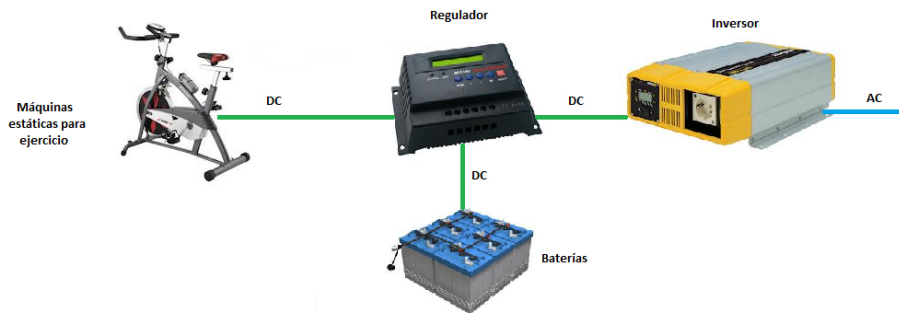
Figura 2. Sistema de generación distribuida en base a bicicletas estáticas aislado a la red [14].
