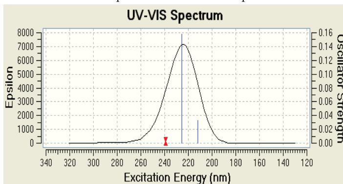
(d) Espectro UV/VIS de S-ibuprofeno
