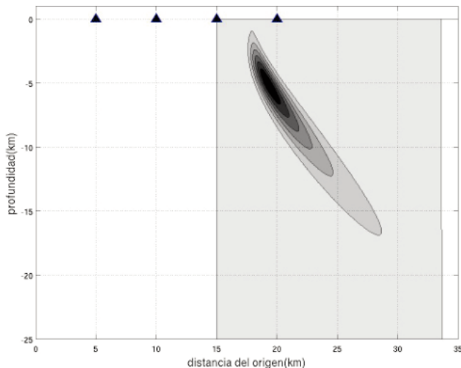
Figura 1 Función de distribución de probabilidad de un terremoto localizado usando cuatro estaciones, son los triángulos en la superficie del terreno. La probabilidad de la posición del sismo es máxima en el color oscuro. La probabilidad de encontrar el sismo en la zona más clara es nula.
