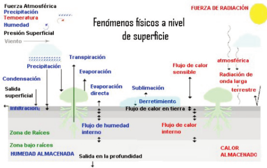
Figura 3 Modelo atmosférico a nivel de superficie, se especifican algunos, de los muchos fenómenos a tomar en cuenta
