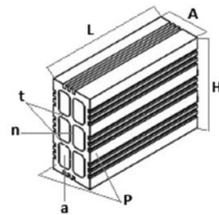
Fig. 2. Dimensiones del Bloque H-10. Fuente: [25]
