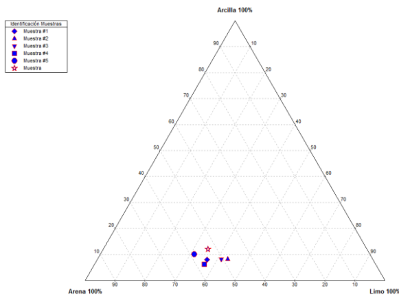
Fig. 6. Graficas de los puntos en el diagrama de Winkler de las arcillas de la empresa. Fuente: Autores.
