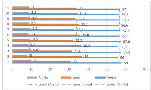
Fig. 9. Tendencias de los resultados del análisis experimental. Fuente: Autores.
