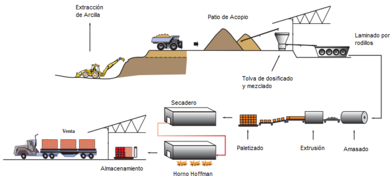
Fig. 1. Esquema de fabricación del bloque. Fuente: [16]
