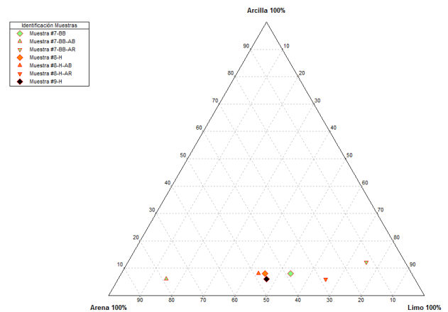
Fig. 8. Graficas de los puntos en el diagrama de Winkler de las arcillas cercanas. Fuente: Autores.
