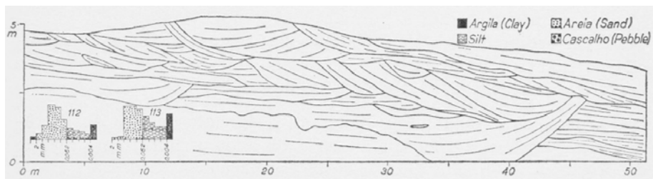
Figura 6 – Estrutura da Formação Guabirotuba, bacia de Curitiba. Corte na rodovia Curitiba-São Paulo (BR2), nas imediações de Quatro Barras. Camadas com estratos cruzados desenvolvidas em dois tipos de sedimentos arenáceo-arcosiano, conforme histogramas. O tipo mais grosseiro salienta-se na erosão diferencial. Ambiente de cones aluviais formados em época semiárida contemporânea à elaboração do pediplano Pd 1
