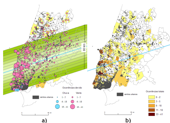
Fig. 12 - Ocorrências devidas ao vento forte e à chuva e totais b) nos dias 23 e 24 de Dezembro de 2010. A linha diagonal mostra a trajectória aproximada do centro da depressão determinada a partir das reanálises NCEP. O espaço delimitado a verde em a) representa um buffer de 40 km para cada lado dessa linha, correspondente à área de maior potencial destruidor da tempestade.
