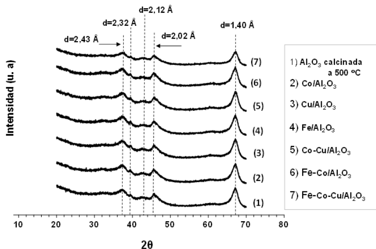
Fig. 4. Difractogramas de rayos X de los catalizadores sintetizados y del soporte catalítico ( \delta -Al 2 O 3 ).
