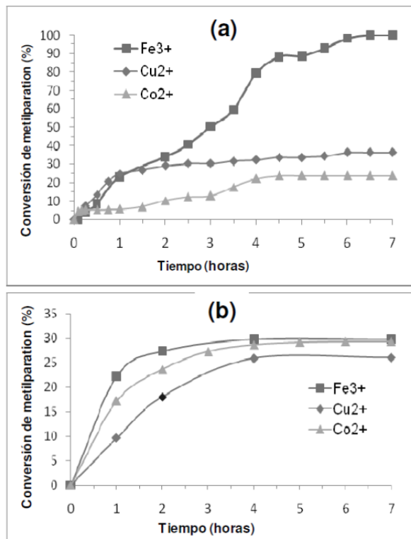
Fig. 6. Degradación catalítica de metilparatión (100 mL a 80 ppm) en medio homogéneo (4 ppm de \text{Fe}^{3+} , \text{Cu}^{2+} o \text{Co}^{2+} ), a presión atmosférica y 25 °C. a) ensayos a pH=3,7 b) ensayos a pH espontáneo (sin control de pH).
