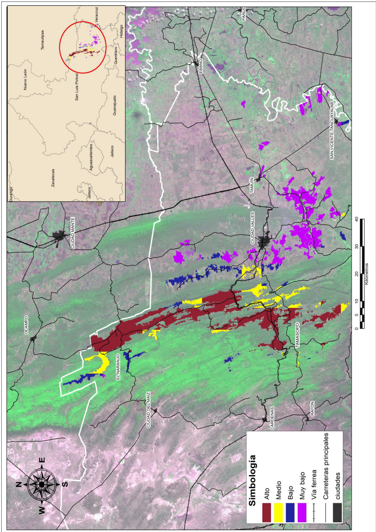
Figura 6. Distribución espacial de la superficie cañera de Huasteca (México) por aptitud al cultivo bajo condiciones de lluvias o secano
