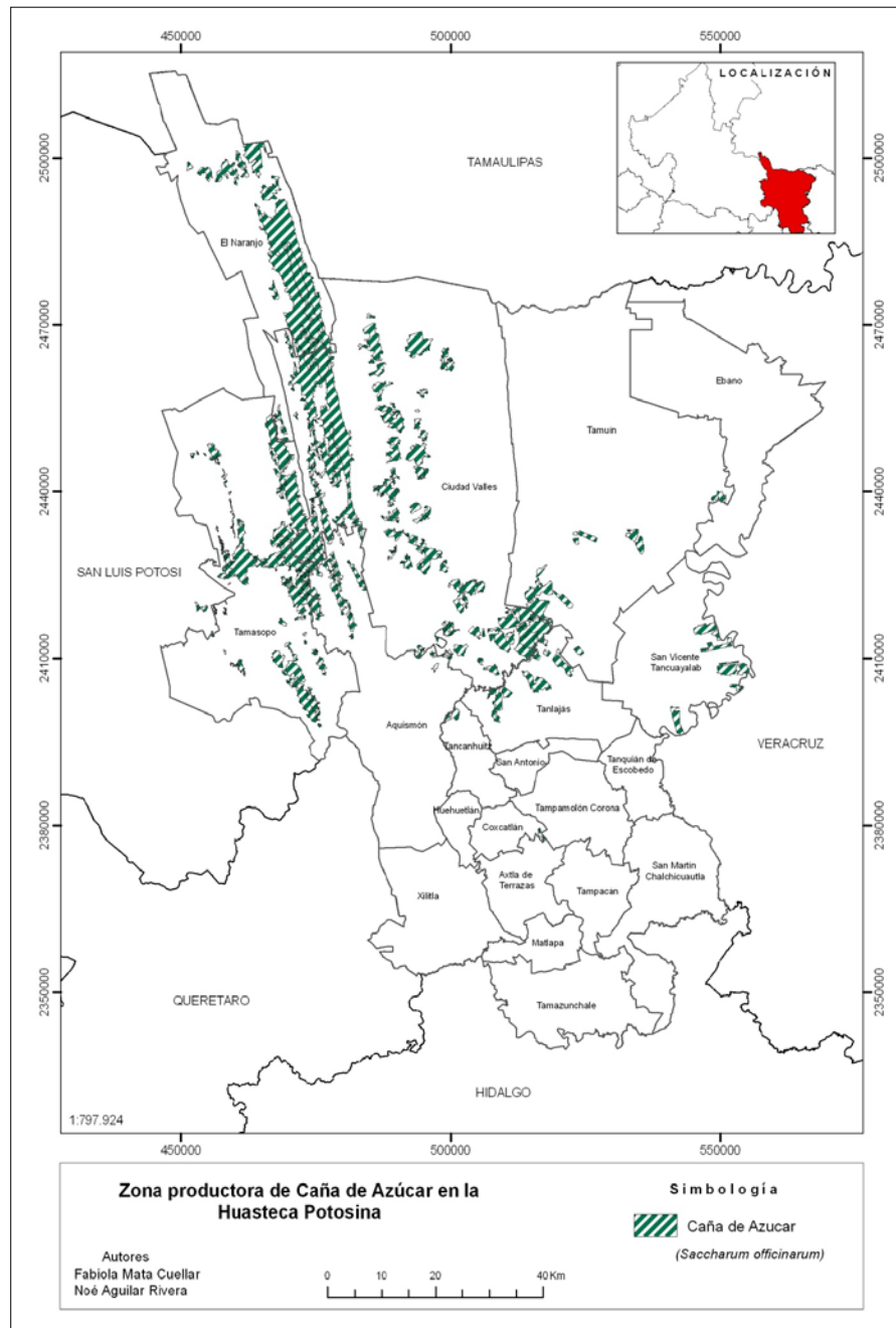
Figura 3. Distribución espacial de la zona cañera de Huasteca (México)
