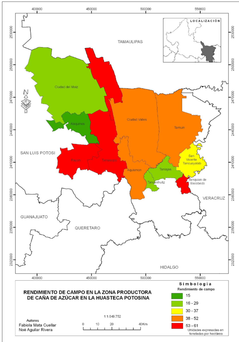
Figura 2. Municipios productores y rendimiento de caña de azúcar en Huasteca (México)
