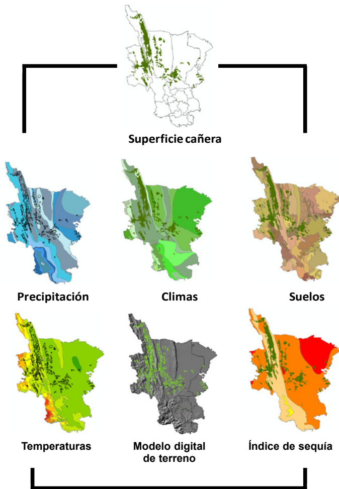
Figura 4. Mapas temáticos empleados en la evaluación de la productividad cañera (escala 1:50.000) Huaste (México)
