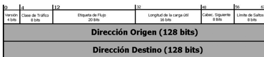
Figura 1. Cabecera IPv6
