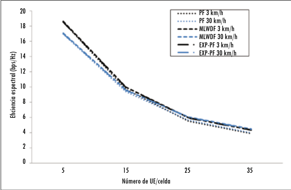
Figura 10. Eficiencia espectral de la red LTE cuando la tasa de codificación de video es de a) 242 kbps y b) 440 kbps
