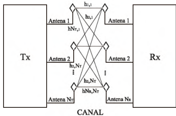
Figura 7. Diagrama en bloques del sistema MIMO (Cortes, 2009).
