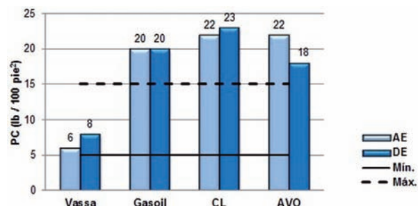
FIGURA 2. Punto cedente de los fluidos evaluados.
