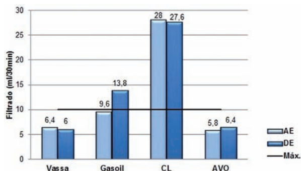
FIGURA 3. Filtrado APAT de los fluidos evaluados.
