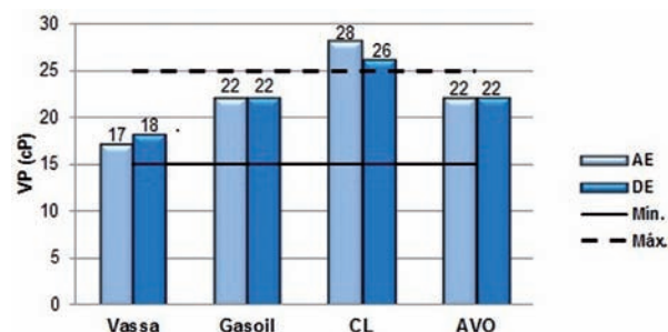
FIGURA 1. Viscosidad plástica de los fluidos evaluados.
