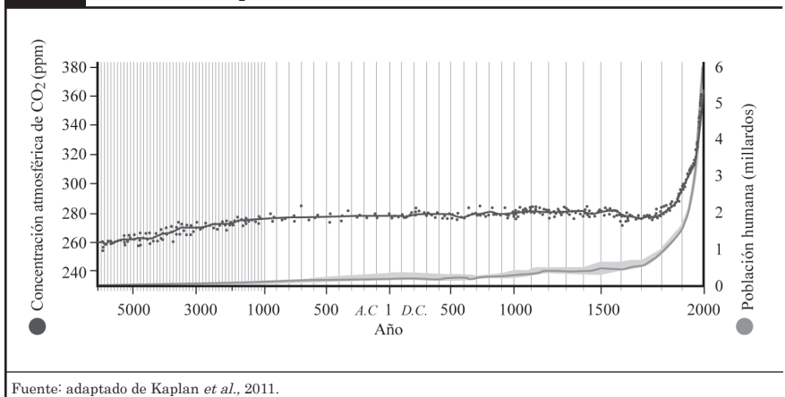
Gráfica 1. Concentración de CO 2 en la atmósfera vs. crecimiento humano.
