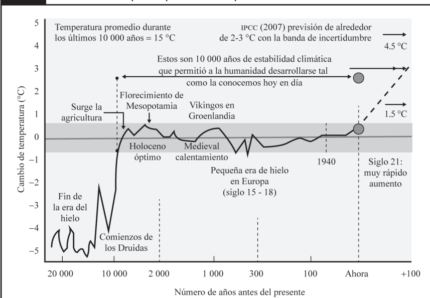
Gráfica 2. Variaciones de la temperatura promedio en la superficie de la Tierra en los últimos veinte mil años.
