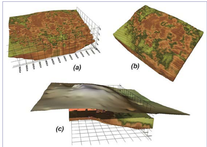
Fig. 4. Construcción del modelo eléctrico 3D-ERT. (a) Se disponen los perfiles espacialmente conforme a su geometría de adquisición. (b) Se interpolan espacialmente las resistividades para formar un modelo compacto tridimensional. (c) Se encaja el modelo eléctrico con el modelo digital del terreno (MDT).
