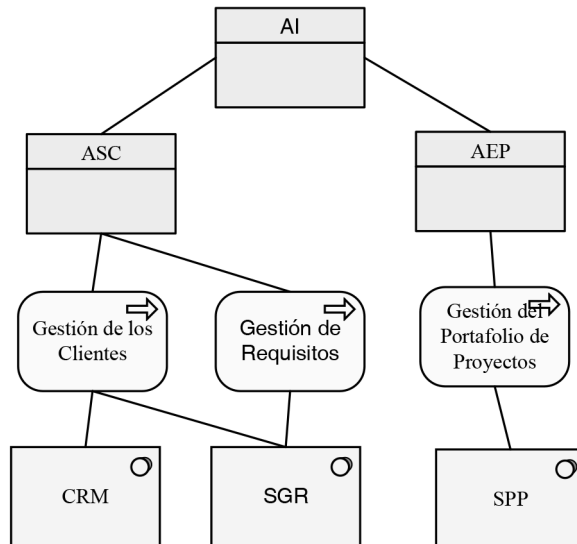
Figura 1 Arquitectura empresarial
