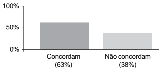
Gráfico 1. Proporção Acordo/Desacordo.
