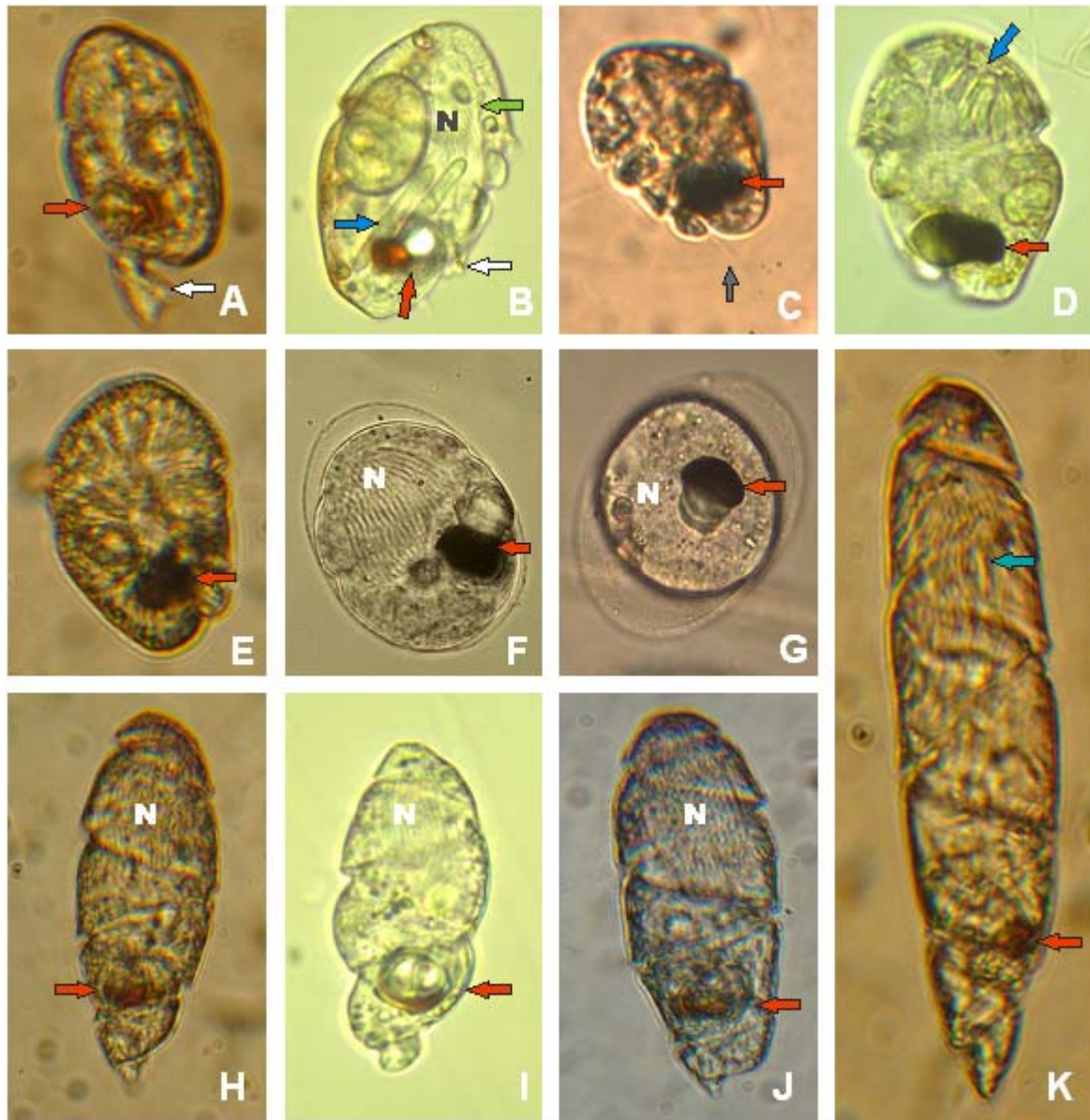
Figure 1: A-K. Microphotographs of 3 species in Bahía de La Paz belonging to the family Warnowiaceae. A. Specimen of Proterythropsis vigilans showing the ocelloid (red arrow), and the posterior extension (white arrow). B. Another specimen of Proterythropsis vigilans showing the ocelloid (red arrow), two extremely large nematocysts (blue arrow), the nucleus (N), several green structures (green arrow), and the posterior extension retracted (white arrow). C-E. Three different specimens of Nematodinium armatum . C. Specimen of Nematodinium armatum showing the ocelloid (red arrow), and the flagellum (gray arrow). D. Specimen of Nematodinium armatum showing the ocelloid (red arrow) and nematocysts (blue arrow). F-G. Pellicle or temporary cysts of Nematodinium (?) showing the ocelloid and the nucleus (N). H-K. Different specimens of Nematodinium torpedo ; red arrows indicate the ocelloid and N the nucleus / A-K. Microfotografías de 3 especies diferentes de la familia Warnowiaceae encontrados en la Bahía de La Paz. A. Espécimen de Proterythropsis vigilans mostrando el oceloide (flecha roja) y el proceso de extensión (flecha blanca). B. Otro espécimen de Proterythropsis vigilans mostrando el oceloide (flecha roja), dos nematocistos extremadamente grandes (flecha azul), el núcleo (N), algunas estructuras verdes (flecha verde) y el proceso de extensión retraído (flecha blanca). C-E. Tres diferentes especímenes de Nematodinium armatum . C. Espécimen de Nematodinium armatum mostrando el oceloide (flecha roja) y el flagelo (flecha gris). D. Espécimen de Nematodinium armatum mostrando el oceloide (flecha roja) y los nematocistos (flecha azul). F-G. Quistes pelliculares o temporales de Nematodinium (?) mostrando el oceloide y el núcleo. H-K. Diferentes especímenes de Nematodinium torpedo ; la flecha roja indica el oceloide y N el núcleo
