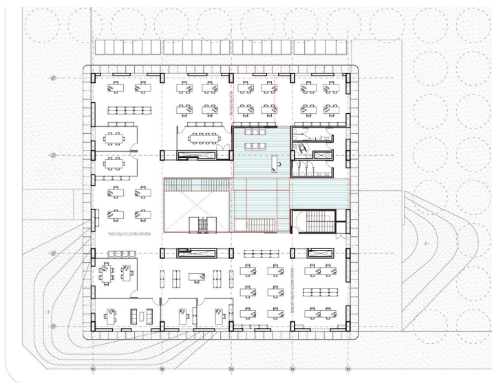
Figura 8. Planta primera. Fuente: COR & Asociados
