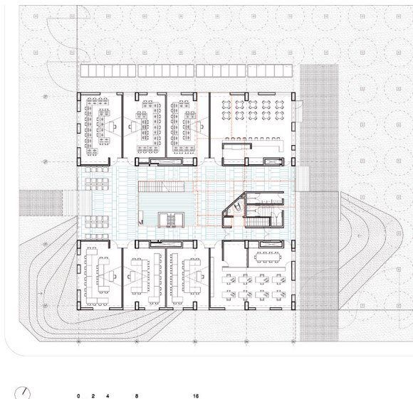
Figura 6. Planta baja. Fuente: COR & Asociados
