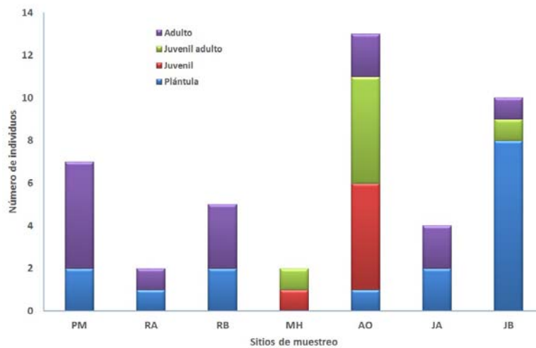
Figura 2. Estructura por estado de Juglans jamaicensis en cada sitio de muestreo.
