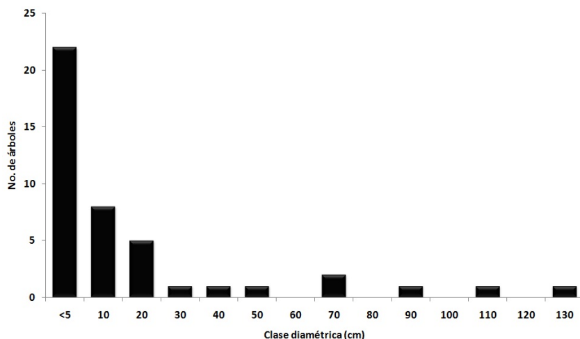
Figura 1. Estructura diamétrica de Juglans jamaicensis en dos unidades zonales de conservación del Parque Nacional Turquino.
