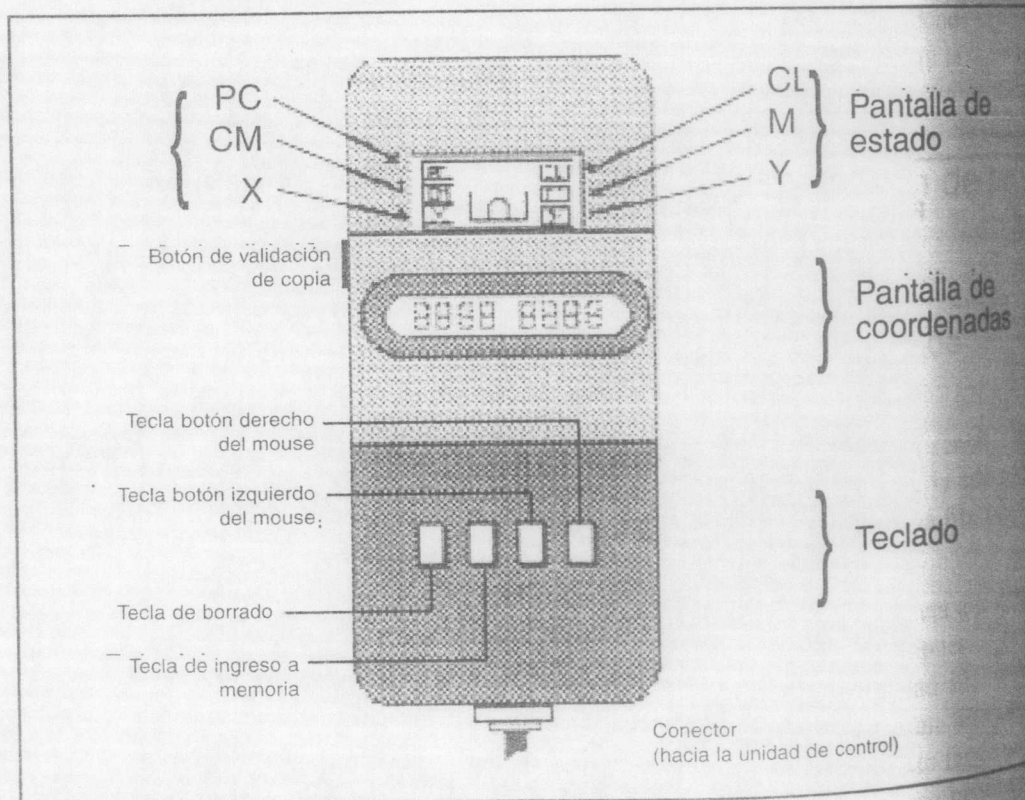
Figura 5 La unidad móvil, sus teclas y pantallas
