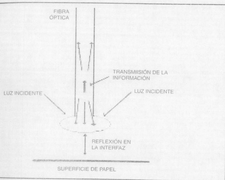
Figura 3 Principio de funcionamiento de la fibra óptica
