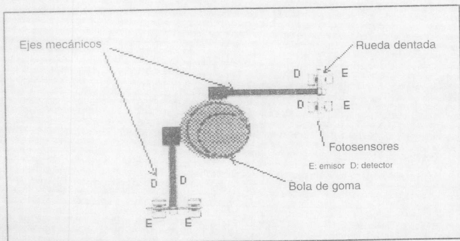
Figura 4 Sistema mecánico de posicionamiento
