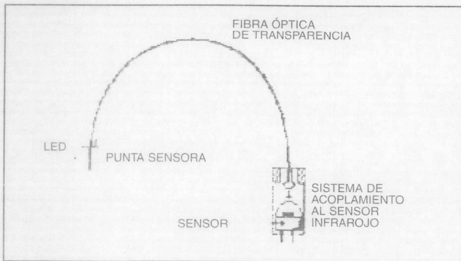
Figura 2 Detalle del acoplamiento de la fibra óptica
