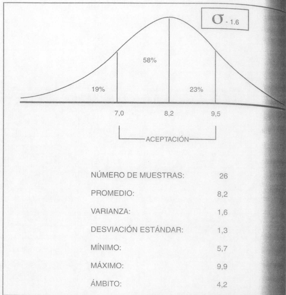
Figura I a Análisis estadístico de los porcentajes de humedad (H) obtenidos
