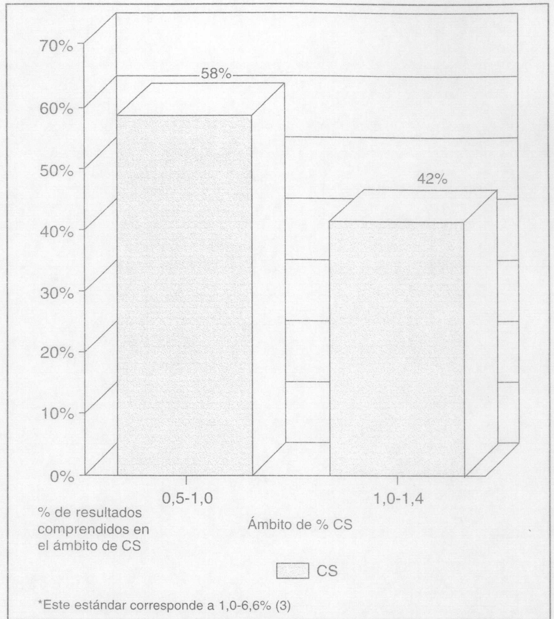
Figura XII Porcentaje de las muestras analizadas que se encuentran dentro y fuera del ámbito* de valores para carbón estándar de maderas tropicales, para contenido de ceniza en base seca (CS)
