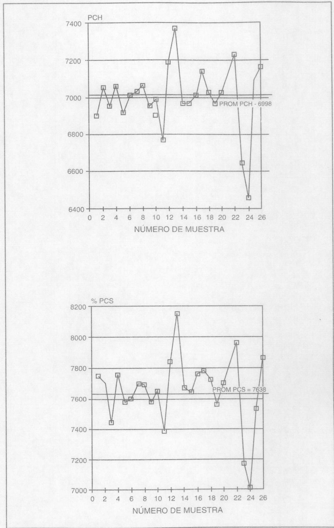
Figura XIII b Valores de poder calórico obtenidos en cada muestra en base húmeda (PCH) y en base seca (PCS)
