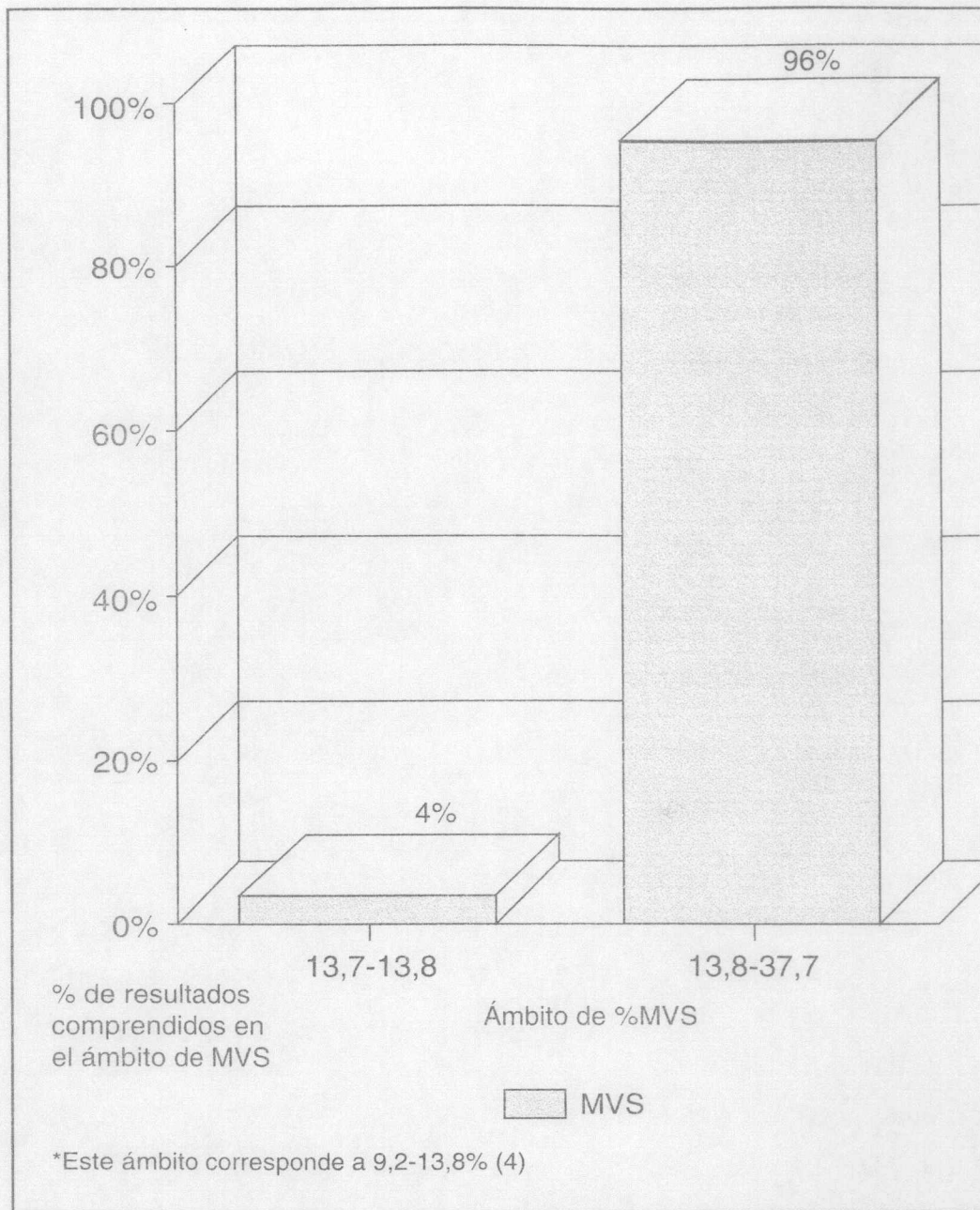
Figura VI Porcentaje de las muestras analizadas que se encuentran dentro y fuera del ámbito de valores encontrados en la literatura para carbón de roble para el contenido de materias volátiles en base seca (MVS)
