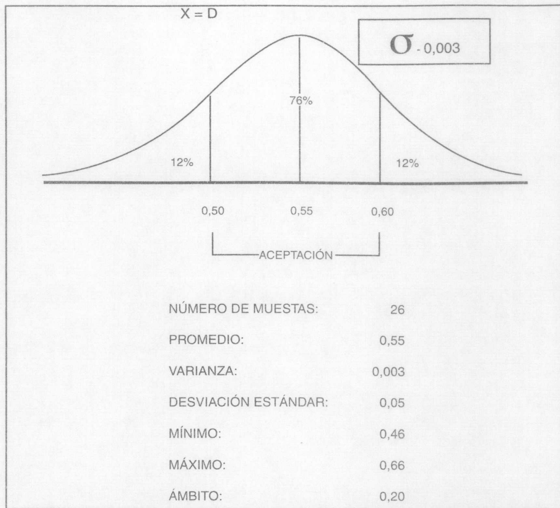
Figura XV a Análisis estadístico de los valores de densidad aparente obtenidos en base seca
