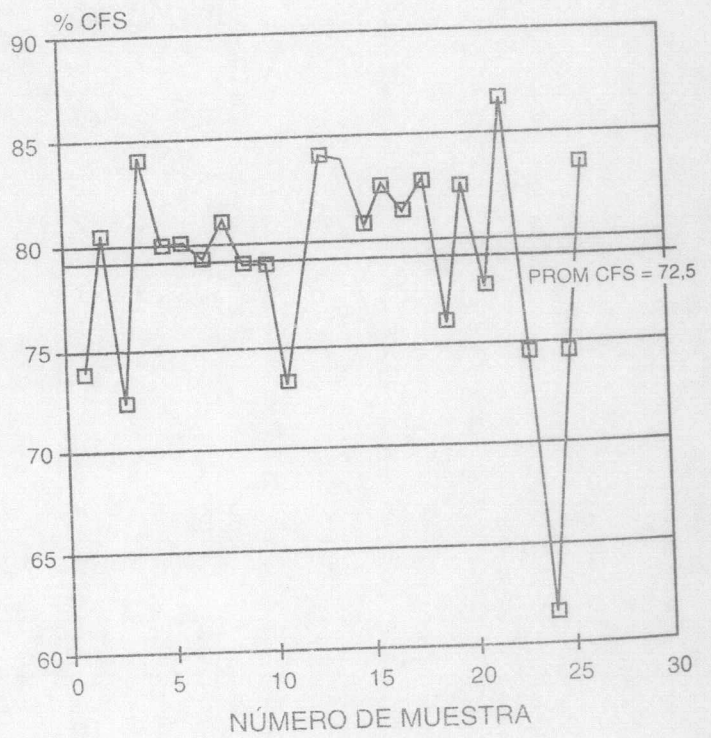
Figura VIIIb Porcentajes de carbono fijo obtenidos en cada muestra en base húmeda (CF) y en base seca (CFS)
