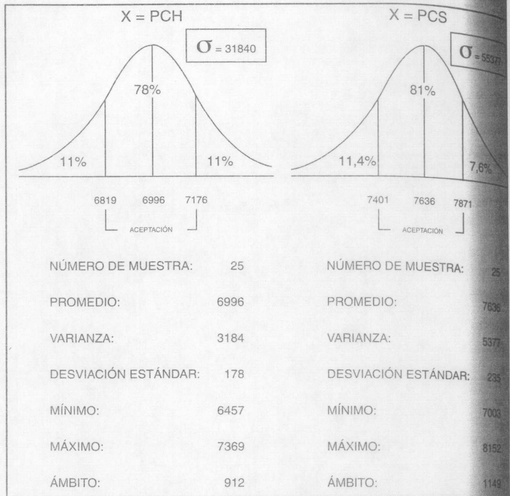
Figura XIII a Análisis estadístico de los valores de poder calórico en base húmeda (PCH) y en base seca (PCS)
