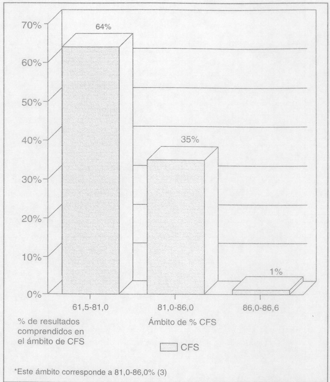
Figura IX Porcentaje de las muestras analizadas que se encuentran dentro y fuera del ámbito* de valores encontrados en la literatura para carbón estándar de maderas tropicales para contenido de carbono fijo, en base seca (CFS)
