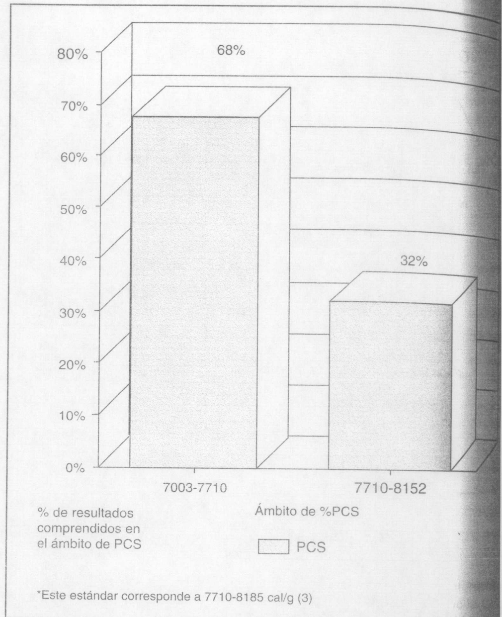
Figura XIV Porcentaje de las muestras analizadas que se encuentran dentro y fuera del ámbito de valores para carbón estándar de maderas tropicales,* para poder calórico en base seca (PCS)
