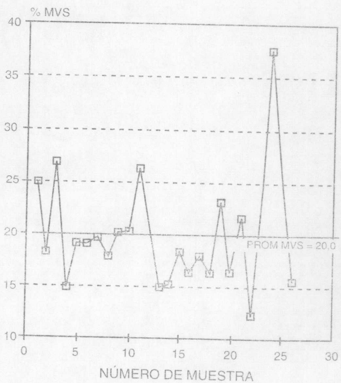
Figura IV b Porcentajes de materias volátiles obtenidas en cada muestra en base húmeda (MV) y en base seca (MVS)
