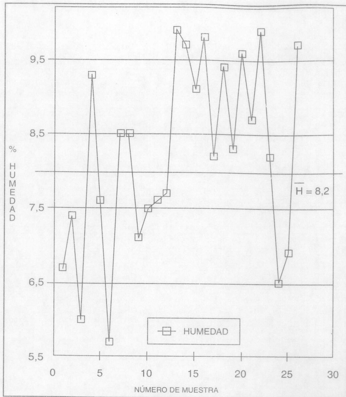
Figura 1 b Porcentaje de humedad obtenido en cada muestra
