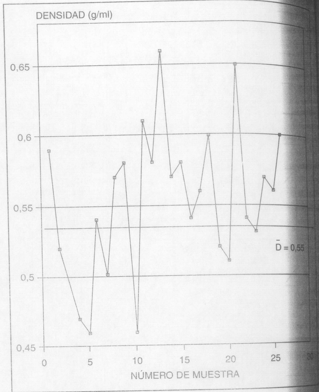
Figura XV b Valores de densidad aparente en base seca (D) obtenidos en cada muestra
