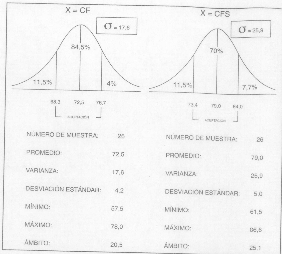
Figura VIII Análisis estadístico de los porcentajes de carbono fijo en base húmeda (CF) y en base seca (CFS)
