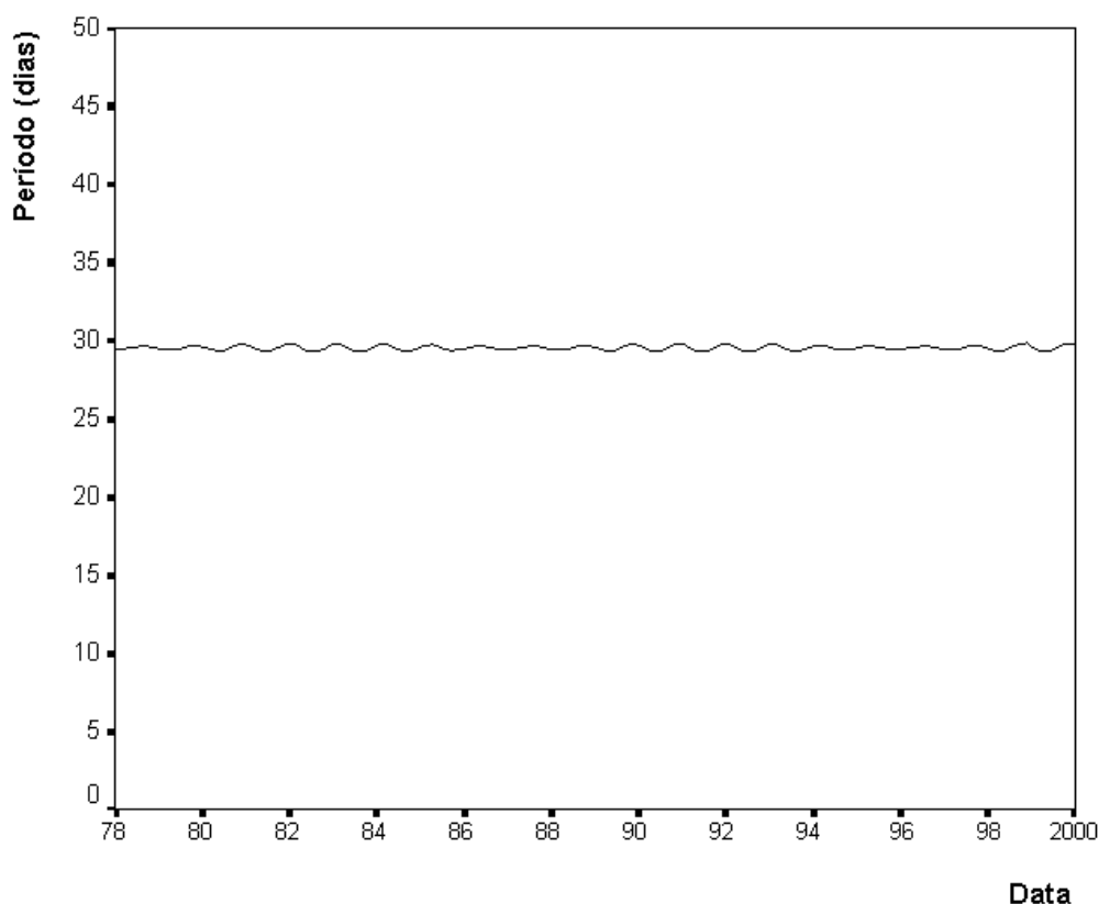
Fig. 1 – Período sinódico da Lua em função do tempo (escala não expandida).
