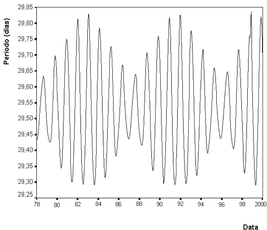
Fig. 2 – Período sinódico da Lua em função do tempo (escala expandida).
