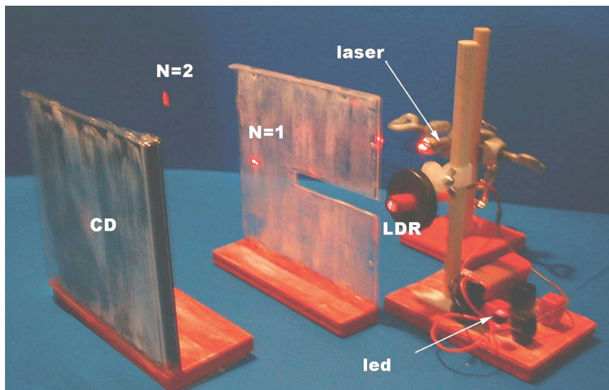
Fig. 14- A figura mostra o espectrofotômetro caseiro construído durante a Oficina, indicando o caráter dual da radiação luminosa.
