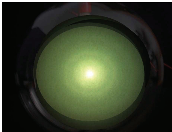
Fig.16- Anéis de difração de elétrons observados na tela fluorescente de uma ampola produzida pela PHYWE (empresa alemã que produz equipamentos didáticos).
