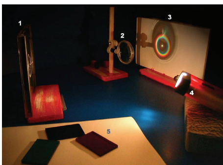
Fig.9- Espectro contínuo produzido por um CD utilizando como fonte de luz uma lanterna, onde: (1) é um CD que decompõe a luz, (2) é uma lupa para projeção do espectro, (3) é o espectro contínuo em forma de anéis, (4) é a lanterna com uma lâmpada de filamento e (5) são filtros, vermelho, violeta e verde.
