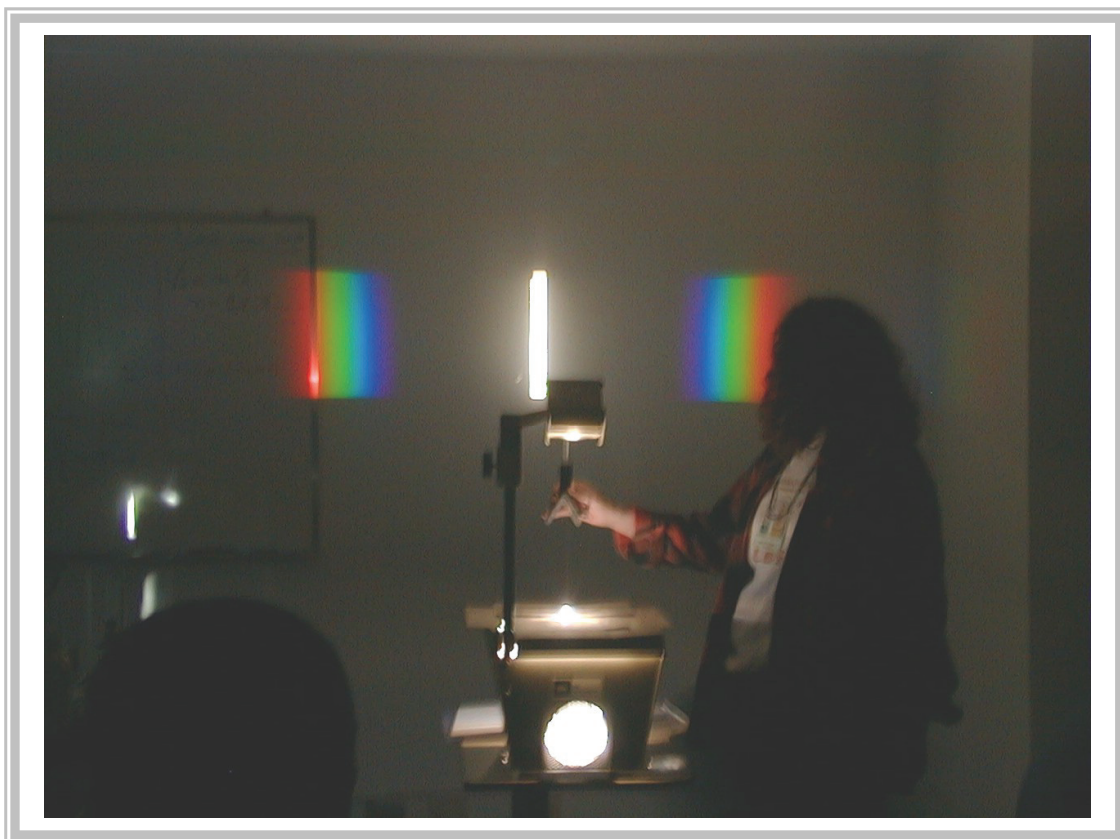
Fig.7- Espectro contínuo obtido utilizando como fonte de luz uma lâmpada de um retroprojetor e uma rede de difração.
