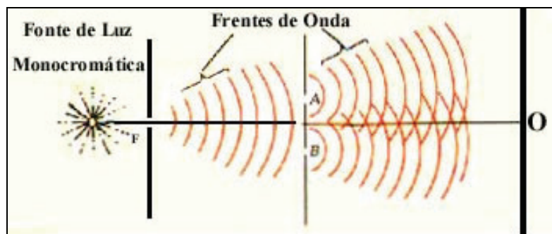
Fig.4- Experiência de Thomas Young.
