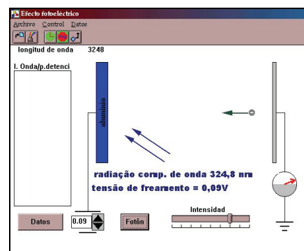
Fig.12- Para se determinar a energia máxima do elétron emitido, devemos aplicar uma diferença de potencial, para frear totalmente o elétron conforme mostra a figura. A energia é proporcional a diferença de potencial aplicada. Software disponível na Internet no Site: http://www.sc.ehu.es/sbweb/fisica/
