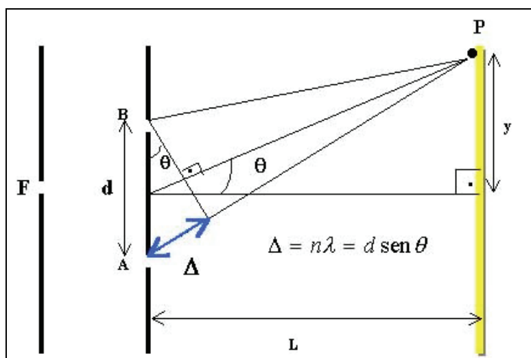
Fig.5- Diagrama esquemático para a determinação do comprimento de onda da luz.
