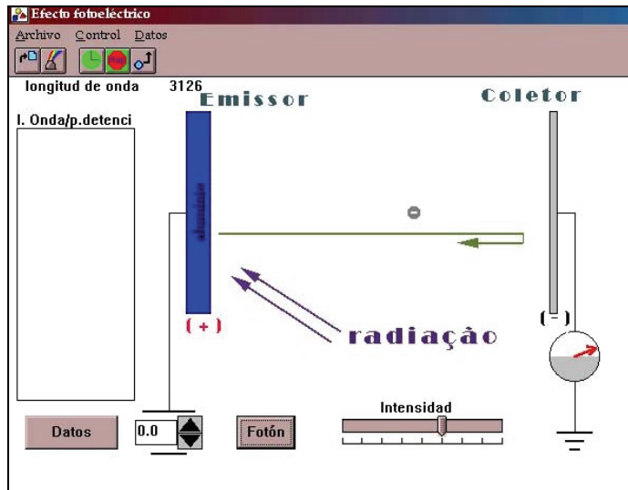
Fig.12- Para se determinar a energia máxima do elétron emitido, devemos aplicar uma diferença de potencial, para frear totalmente o elétron conforme mostra a figura. A energia é proporcional a diferença de potencial aplicada. Software disponível na Internet no Site: http://www.sc.ehu.es/sbweb/fisica/
