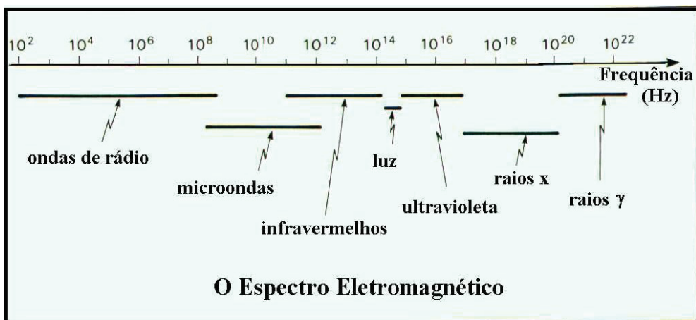
Fig.2- Espectro eletromagnético, mostrando os diferentes tipos de ondas eletromagnéticas e os correspondentes valores de freqüência.
