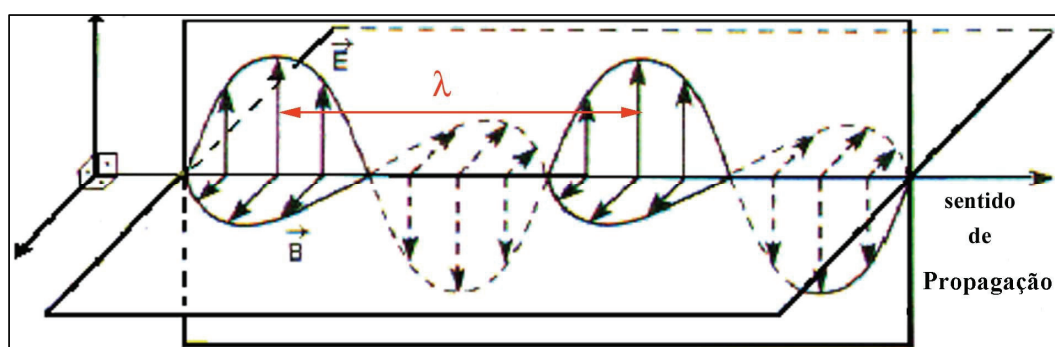
Fig.1- Representação esquemática de uma onda eletromagnética, mostrando os vetores campo elétrico e magnético, bem como o comprimento de onda.
