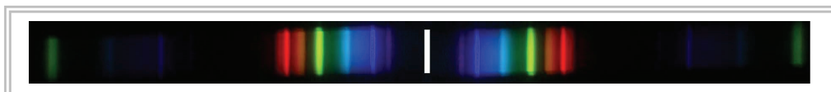
Fig.8- Espectro de uma lâmpada fluorescente de mercúrio, mostrando algumas linhas características deste gás.
