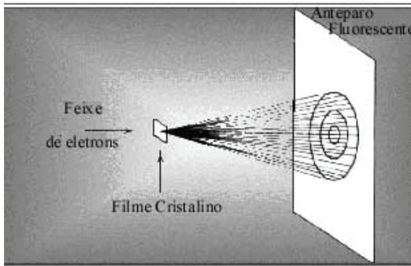
Fig.15- Esquema do experimento de G.P Thomson para a difração de elétrons; um feixe de elétrons incide em um fino cristal produzindo anéis de interferência na tela
