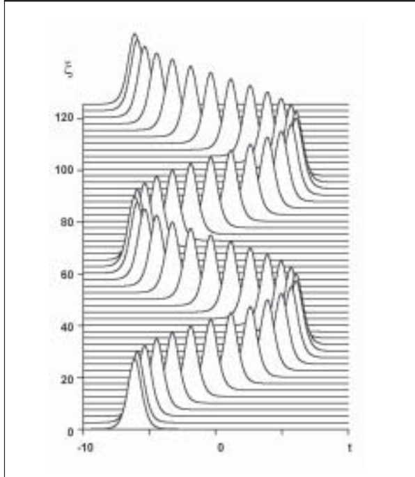
Figura 2. Dinámica no lineal del solitón de la ecuación de Gross Pitaevskii en un potencial armónico. Aquí por \tau se entiende el eje espacial y a \xi se considera como el eje temporal (Hernandez et al. , 2005).
