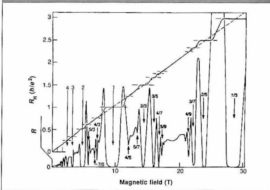
FIGURA 1. LA LINEA DIAGONAL PUNTEADA REPRESENTA LA RESISTENCIA CLÁSICA DE HALL Y LA LINEA GRUESA ESCALONADA LOS RESULTADOS EXPERIMENTALES. LOS CAMPOS MAGNÉTICOS QUE CAUSAN LOS ESCALONAMIENTOS ESTÁN MARCADOS CON FLECHAS. NÓTESE PARTICULARMENTE EL ESCALON DESCUBIERTO POR STORMER Y TSUI CON EL PARÁMETRO DE LLENADO f = 1/3 ; EL ALTO VALOR DEL CAMPO MAGNÉTICO, Y LOS PLATOS DESCUBIERTOS POR VON KLITZING (CON PARÁMETROS DE LLENADO ENTEROS CON CAMPOS MAGNÉTICOS DÉBILES) (SCIENCE, 1990).
