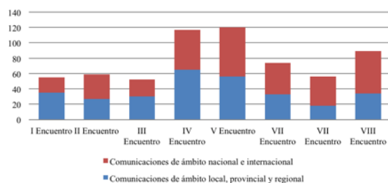
Grafico 2. Comparación del ámbito de estudio de las comunicaciones presentadas a los Encuentros de Investigadores del franquismo (1992-2013)
