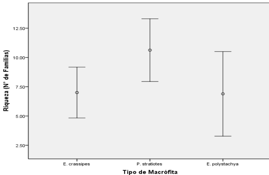
Figura 03. Riqueza de familias de macroinvertebrados acuáticos asociados a tres macrófitas en la laguna de Moronacocho (Iquitos- Perú).
