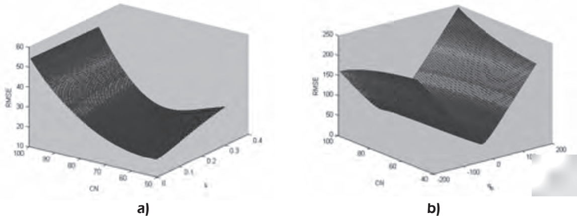
Figura 7. Identificación de los espacios del modelo. a) Relación entre los parámetros CN y k . b) Relación entre los parámetros CN y Q_b .
