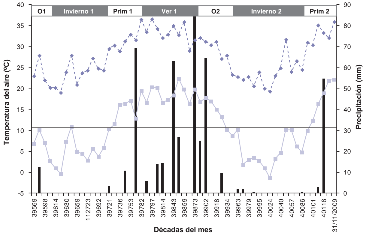
Figura 2. Dinámica temporal de la precipitación (mm, barras) y de temperaturas máxima (rombos) y mínima (cuadrados) del aire (°C, promedio decádico). Período experimental 2008-09, campo experimental La María, INTA EEA Santiago del Estero. Abreviaturas: O, otoño; Prim, primavera; Ver: Verano.
