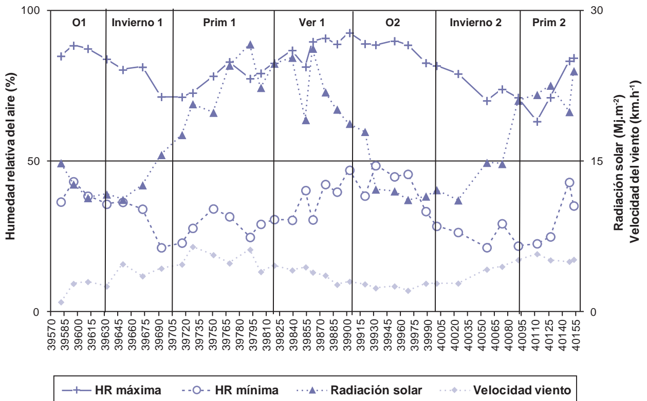
Figura 3. Dinámica temporal de los promedios de la humedad relativa del aire máxima (cruces) y mínima (círculos), la radiación solar (triángulos) y la velocidad del viento a 2 m de altura (rombos) observadas entre fechas de muestreo. Período 2008-09, campo experimental La María, INTA EEA Santiago del Estero. Abreviaturas: O, otoño; Prim, primavera; Ver: Verano.
