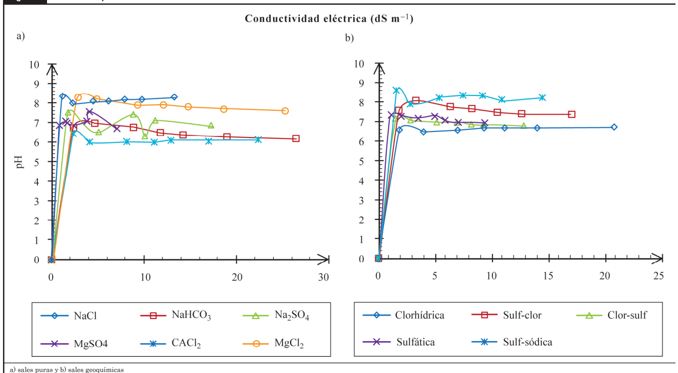
Figura 2. Relación del pH con la conductividad eléctrica.
