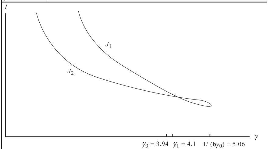
Figura 4. Gráfica de las funciones J_i . Nótese que se intersectan en \gamma_1 \approx 4.1 > \gamma_0 \approx 3.94 . Valores de los parámetros a = 0.4 , b = 0.05 .
