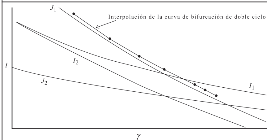
Figura 6. La figura muestra la interpolación geométrica de la curva de bifurcación de ciclos a partir de puntos estimados mediante un programa gráfico ex profeso . Los valores de los parámetros son a = 0.5, b = 0.01 , los intervalos de los parámetros \gamma e I son: 3.94 < \gamma < 5.68, 0.13 < I < 0.82 respectivamente.
