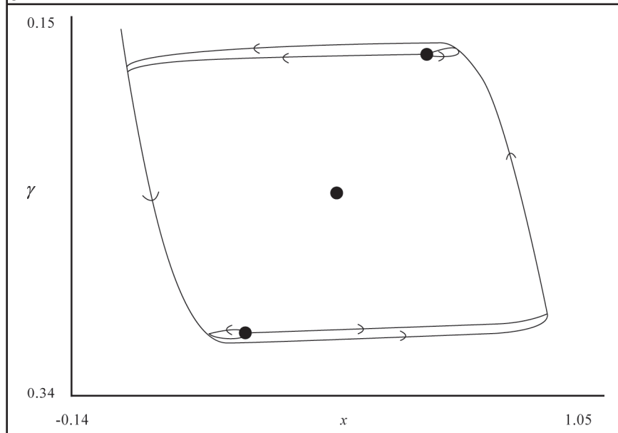
Figura 2. En esta figura se muestran tres equilibrios, una silla y dos nodos. Ambos nodos son inestables.
