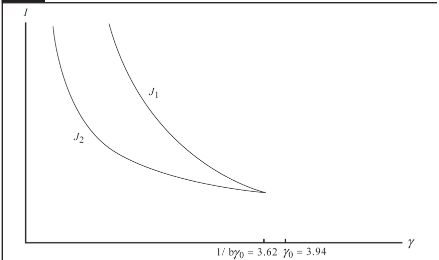
Figura 3. Gráfica de las funciones J_i .
