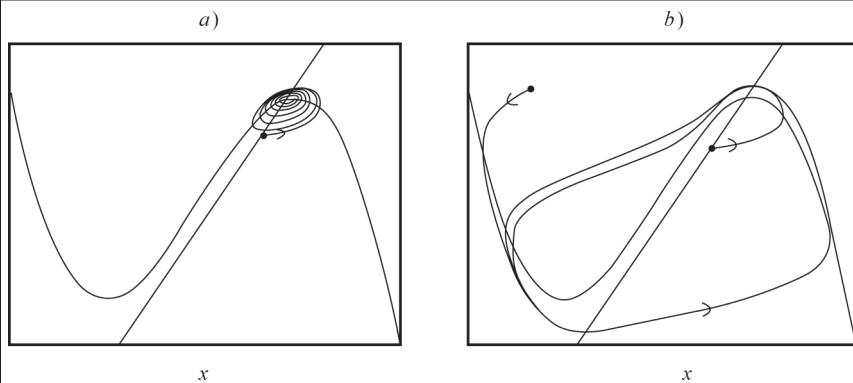
Figura 5. Coexistencia de un equilibrio estable y un ciclo límite estable en el plano fase del sistema FHN.
