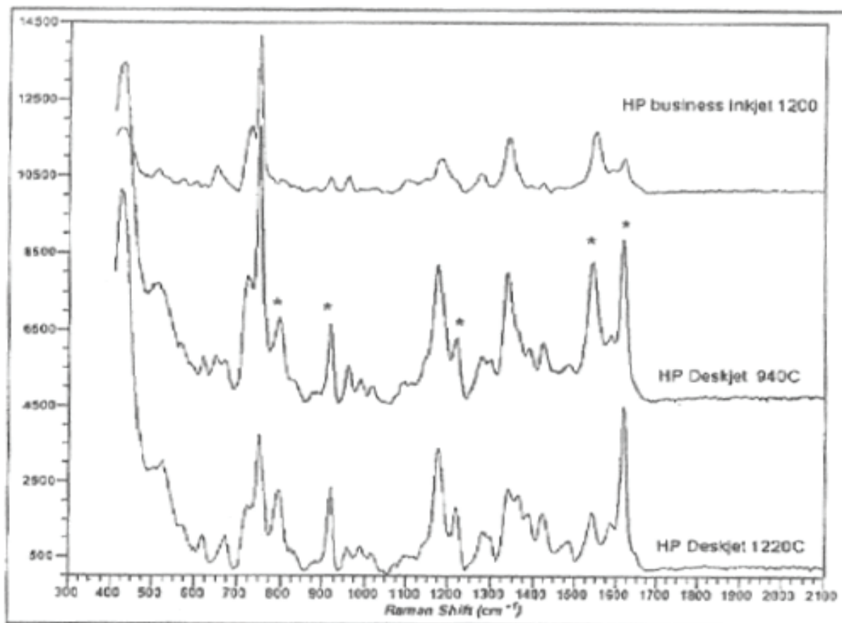
Fig. 2. Espectros Raman obtenidos de tintas de tres impresiones inkjet con el equipo Forum. Fuente: Ezcurra Gondra, Magdalena, Grávalos, Goyo R., op cit, pag. 227
