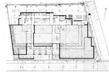
[Fig. 14] Mies, Casa con tres patios (1935). Casa Huarte. Planta baja.
