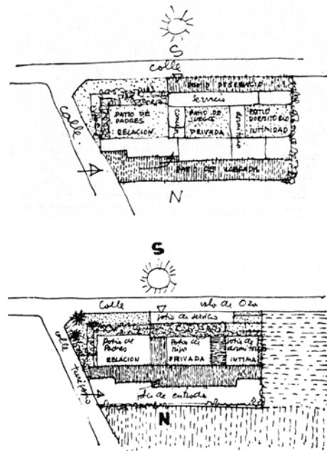
[Fig. 3] Casa Huarte. Croquis dibujados por Molezún donde aparecen sombreados alternativamente llenos y vacíos.
