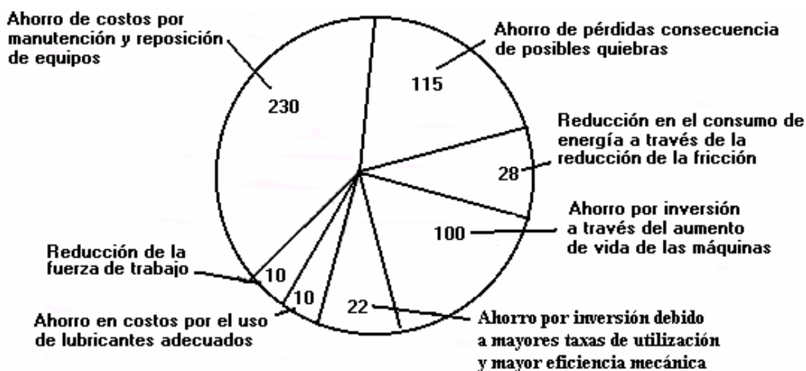
Figura 1. Ahorro resultante debido al empleo de conceptos de tribología. Los valores están expresados en millones de libras esterlinas (valores a 1966) [6]
