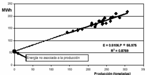
Figura 6. Diagrama de consumo Electricidad Vs producción.
